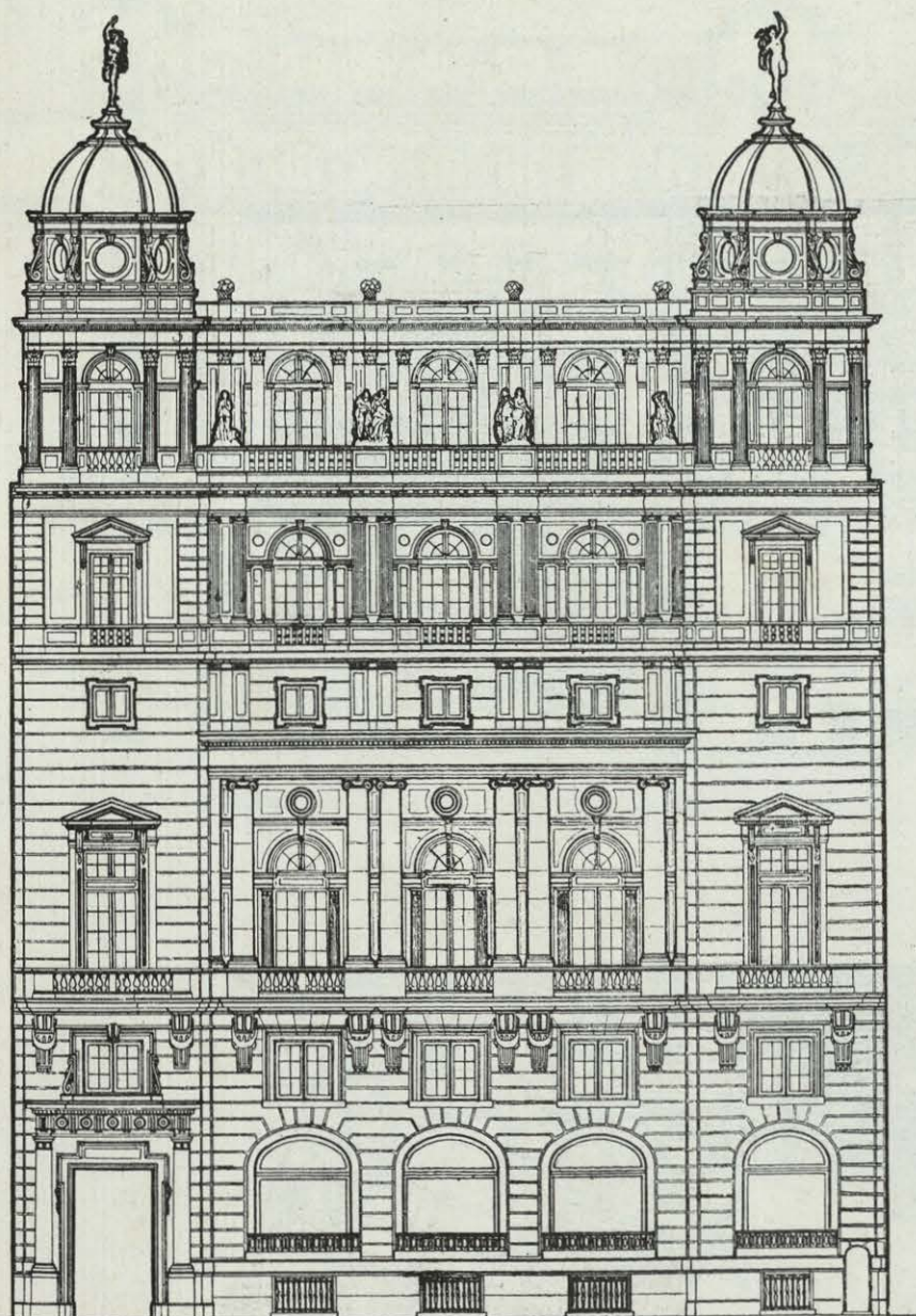
FACHADA PRINCIPAL.
