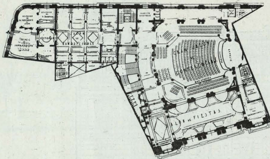
FLANTA PRINCIPAL.
